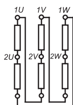
Схема обмотки
