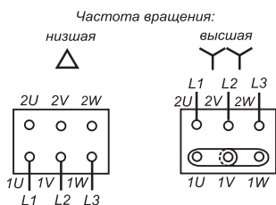
Схема соединений на панели
