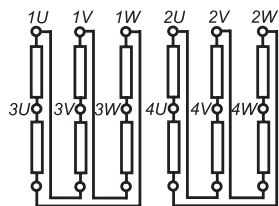
Схема обмотки
